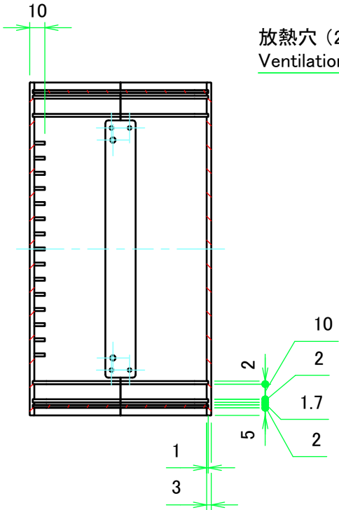
B-B ( 1 : 3.5 )
