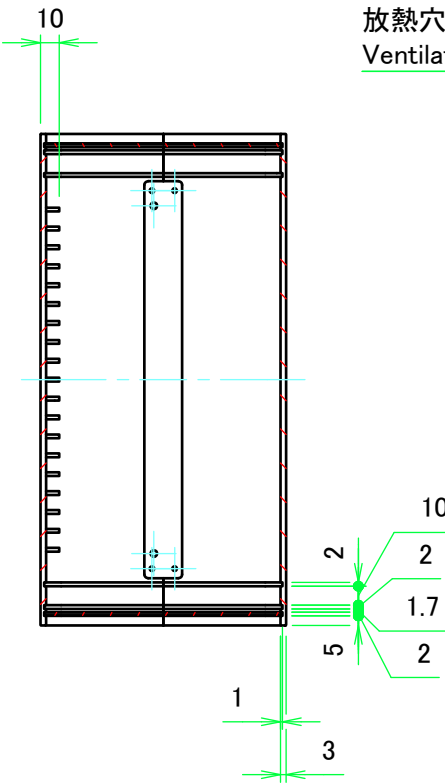
B-B ( 1 : 4 )
