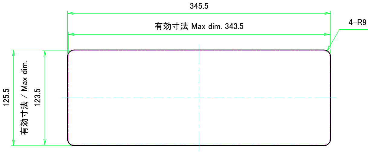
パネル表面 / Panel Frontside
