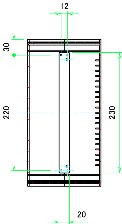
A-A ( 1 : 4.5 )
