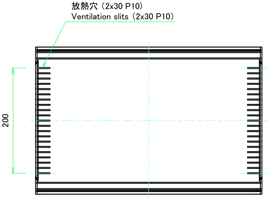
上カバー(内視) Top cover (Internal view)
