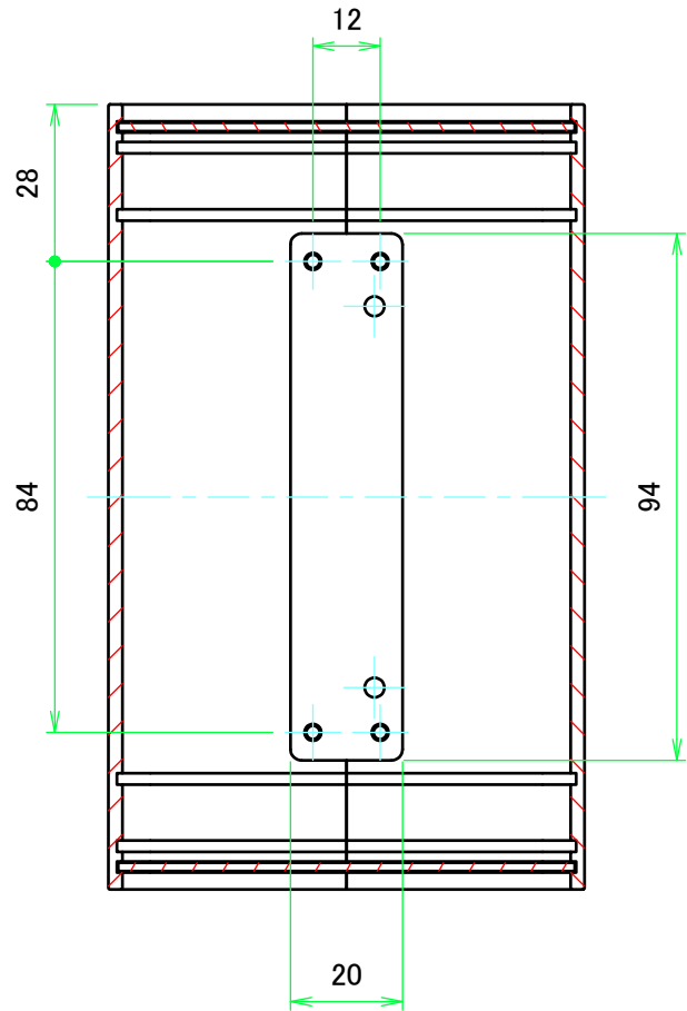
A-A ( 1 : 1.5 )
