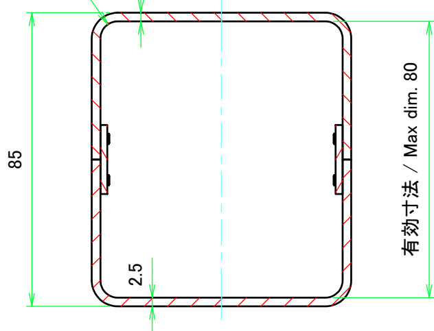
4-R5 D-D ( 1 : 1.5 )
