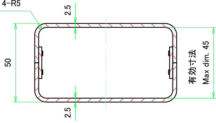
D-D ( 1 : 1.5 )
