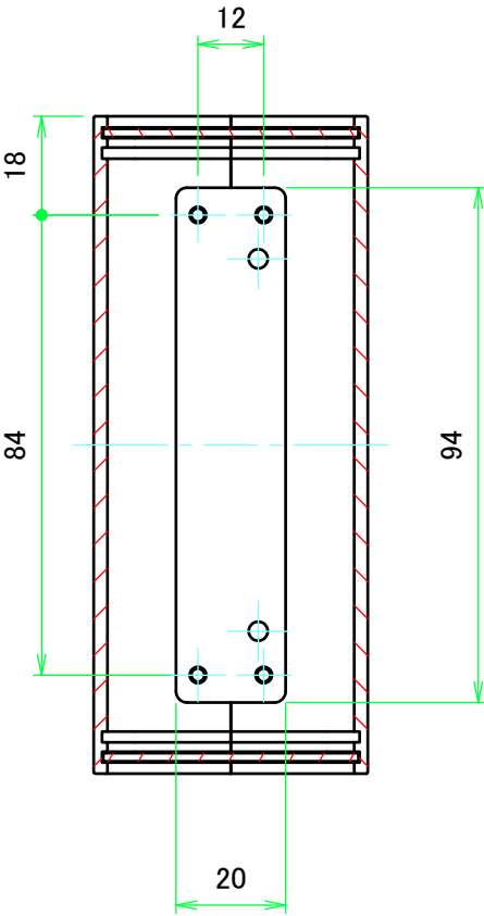
A-A ( 1 : 1.5 )
