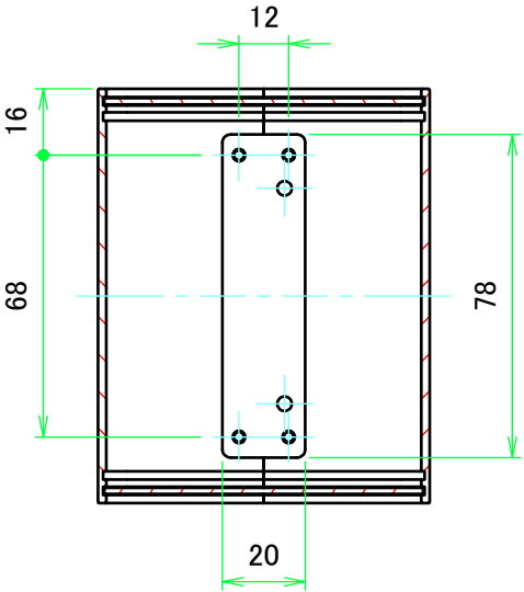
A-A ( 1 : 2 )
