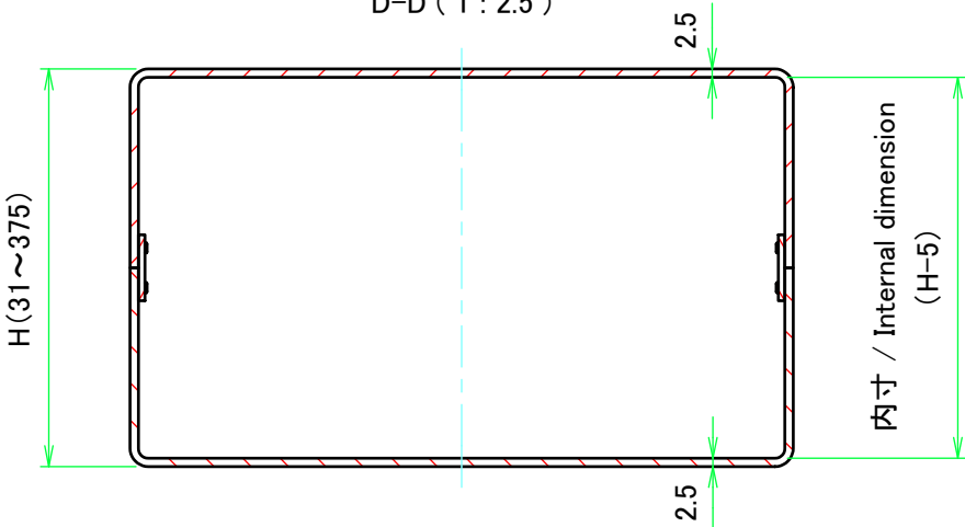
D-D ( 1 : 2.5 )
