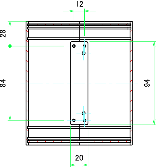
A-A ( 1 : 2.5 )
