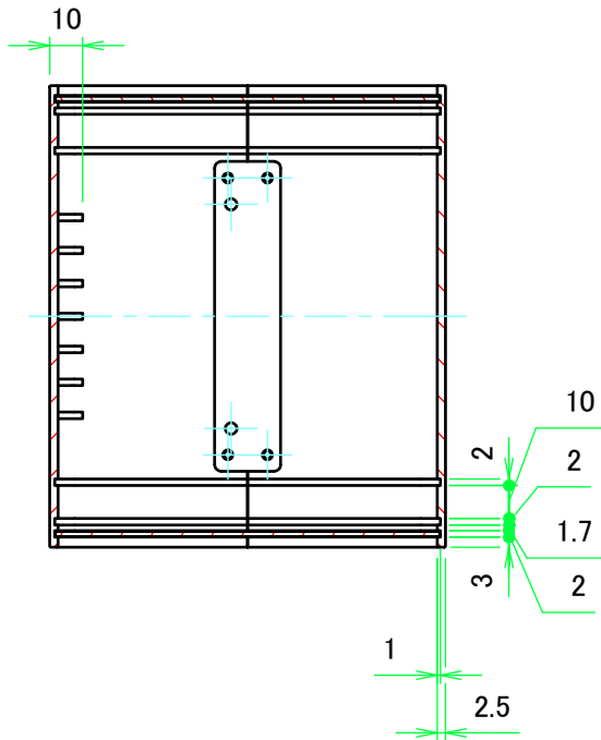
B-B ( 1 : 2.5 )
