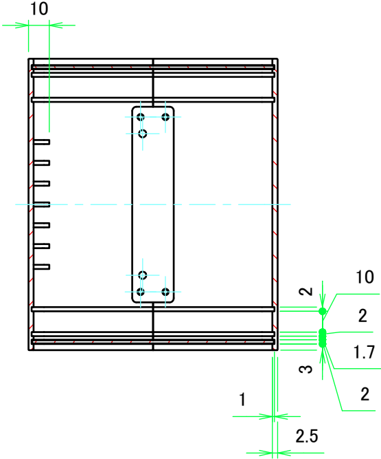
B-B ( 1 : 2.5 )
