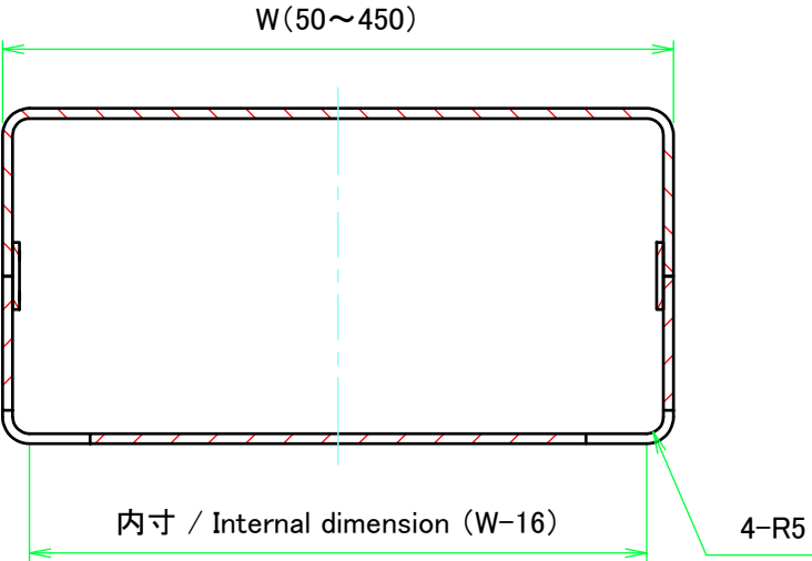
C-C ( 1 : 2.5 )
