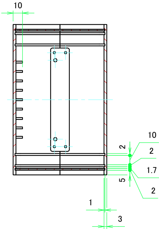
B-B ( 1 : 2.5 )
