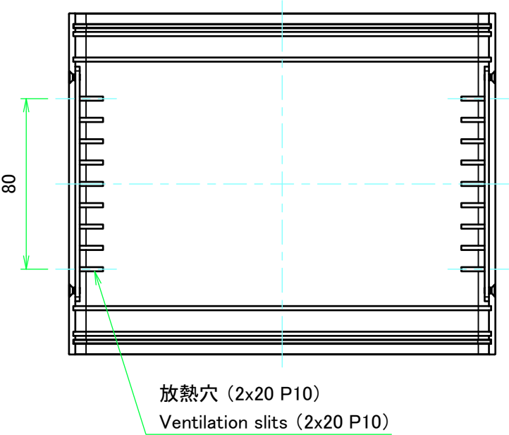
上カバー(内視) Top cover (Internal view)
