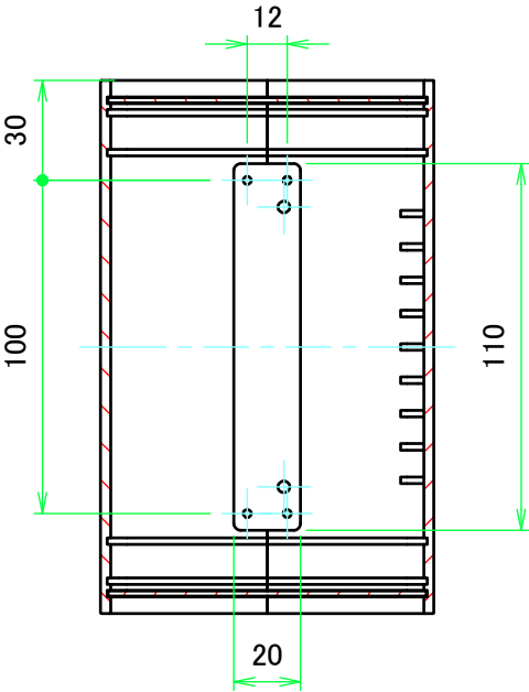
A-A ( 1 : 2.5 )
