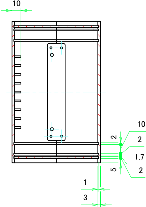
B-B ( 1 : 2.5 )
