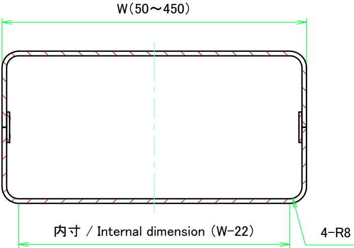
C-C ( 1 : 2.5 )
