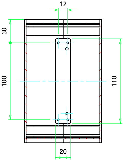
A-A ( 1 : 2.5 )
