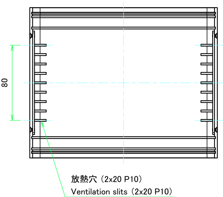
上カバー(内視) Top cover (Internal view)
