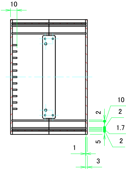
B-B ( 1 : 3 )
