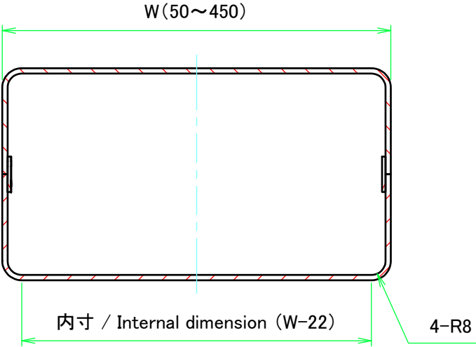
C-C ( 1 : 3 )
