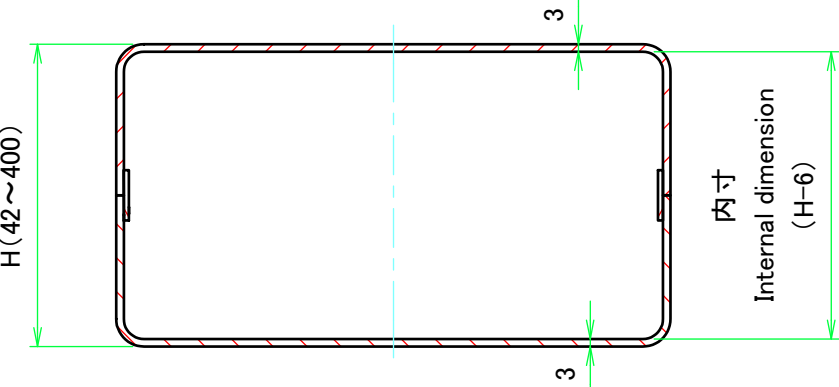
D-D ( 1 : 3 )
