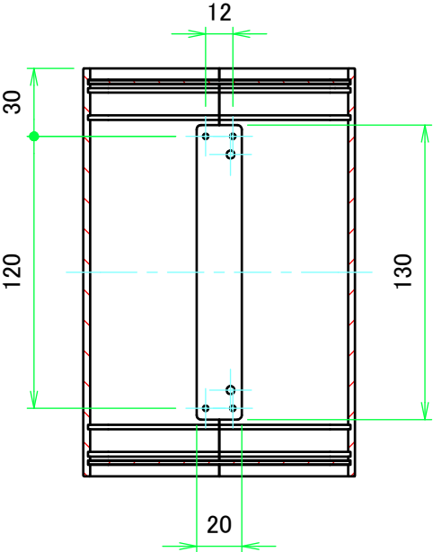
A-A ( 1 : 3 )
