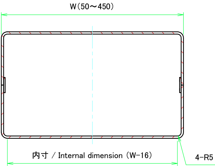
C-C ( 1 : 3 )
