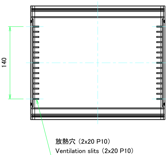
上カバー(内視) Top cover (Internal view)
