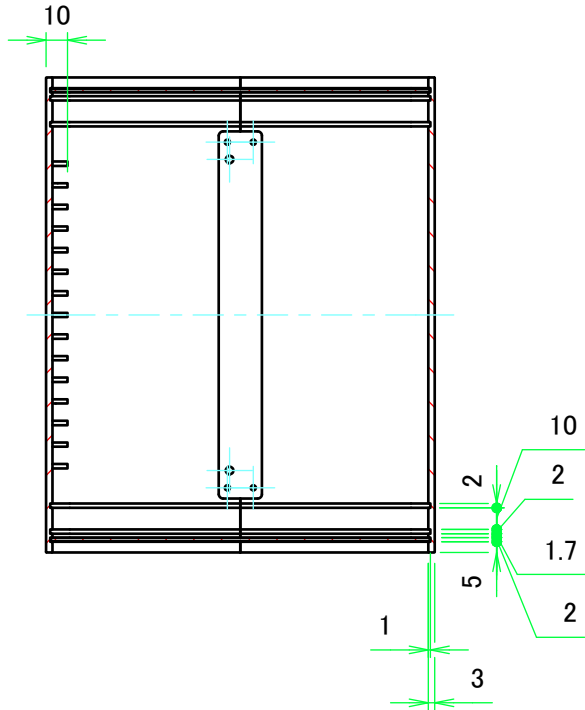
B-B ( 1 : 3.5 )
