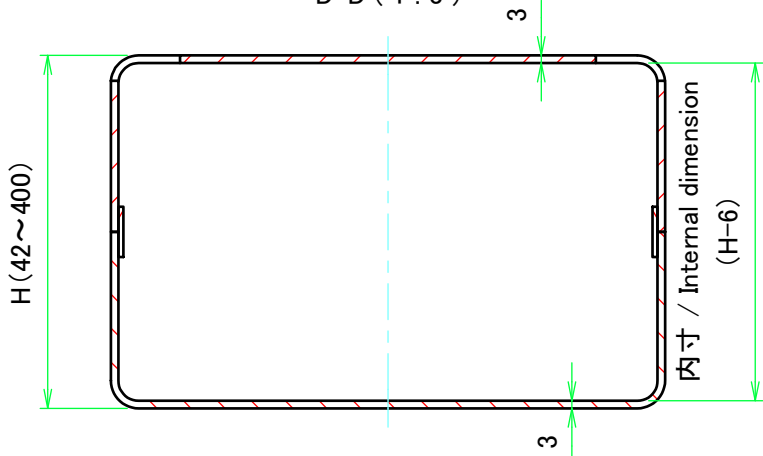
D-D (1:3)
