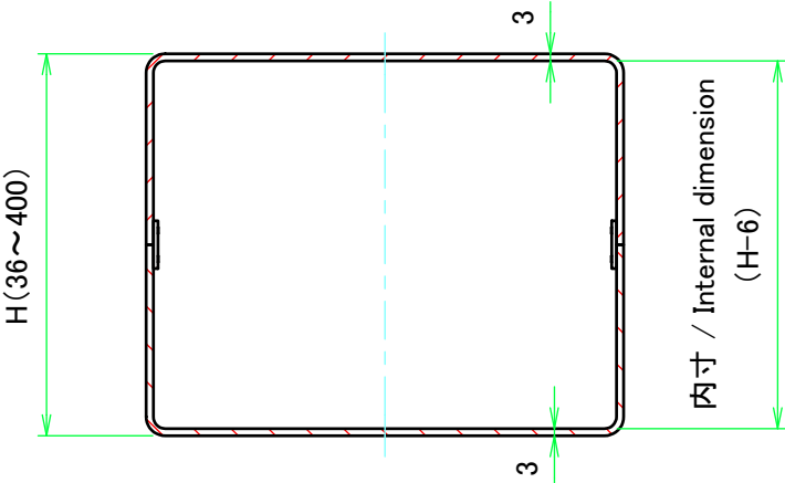
D-D ( 1 : 3.5 )
