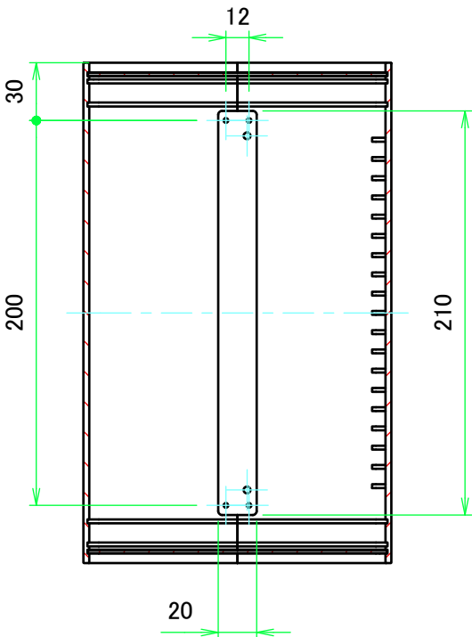
A-A ( 1 : 3.5 )
