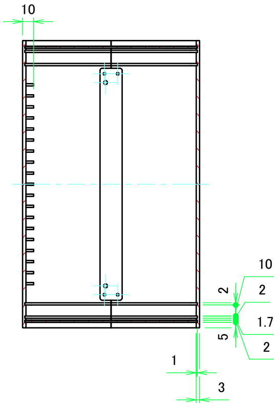
B-B ( 1 : 3.5 )
