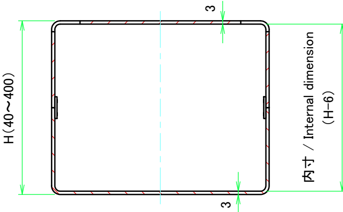
D-D ( 1 : 3.5 )
