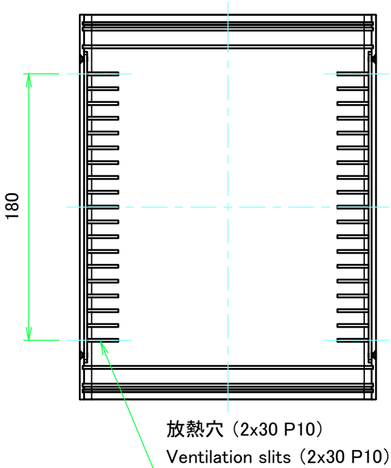
上カバー(内視) Top cover (Internal view)
