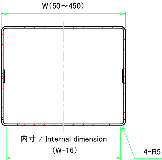
C-C ( 1 : 3.5 )
