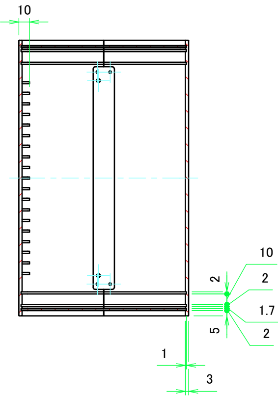
B-B ( 1 : 3.5 )
