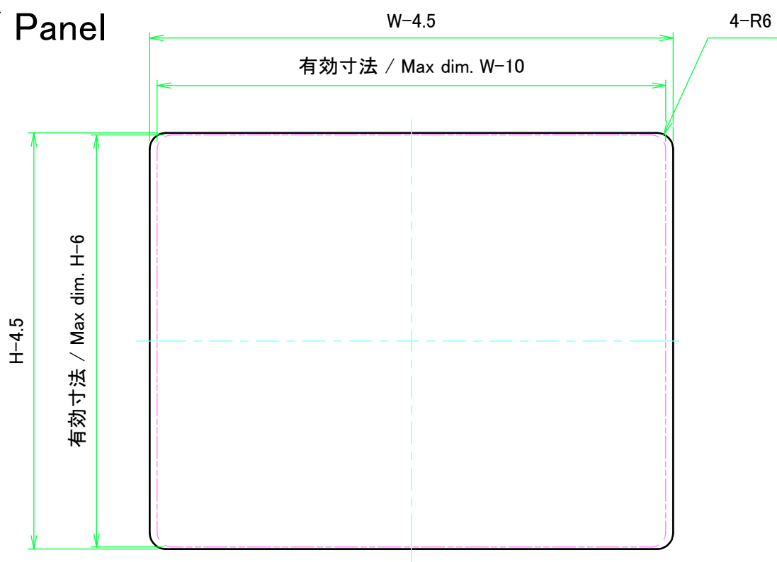
パネル表面 / Panel Frontside
