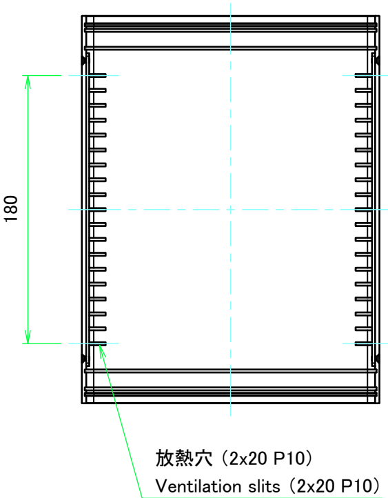
上カバー(内視) Top cover (Internal view)
