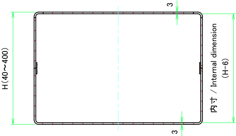
D-D ( 1 : 4 )
