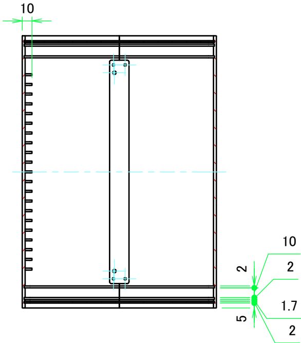
B-B ( 1 : 4 )
