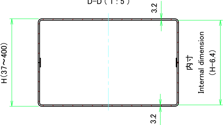
D-D ( 1 : 5 )
