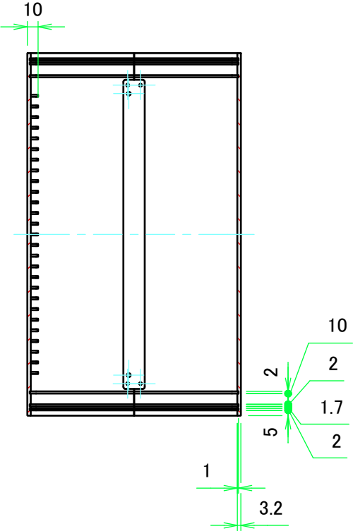
B-B ( 1 : 5 )
