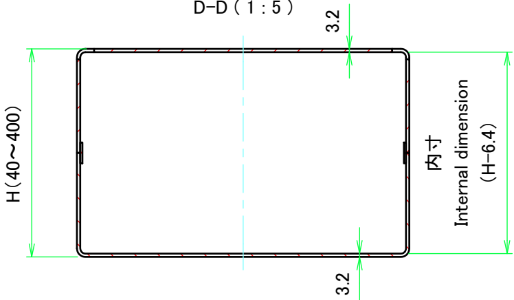
D-D ( 1 : 5 )
