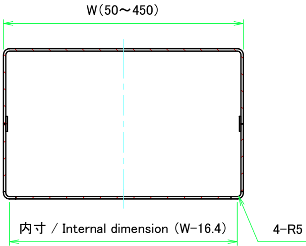
C-C ( 1 : 5 )
