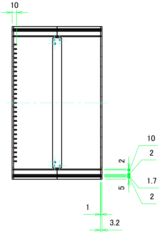
B-B ( 1 : 5 )
