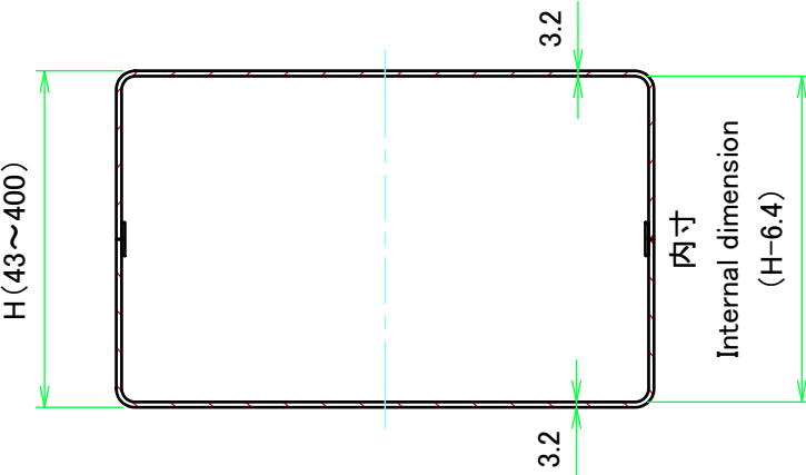
D-D (1:5)
