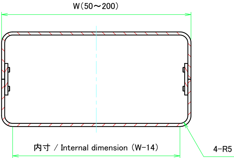
C-C ( 1 : 1.5 )
