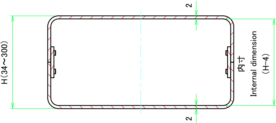
D-D ( 1 : 1.5 )
