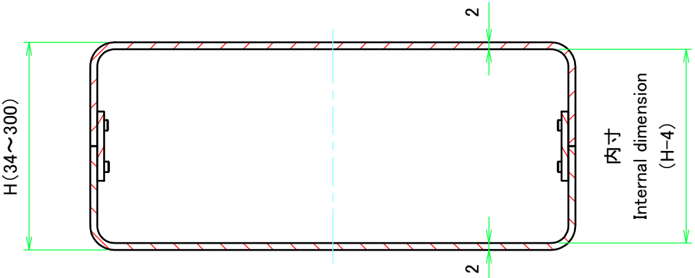
D-D ( 1 : 1.5 )
