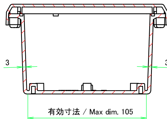
B-B ( 1 : 2 )
