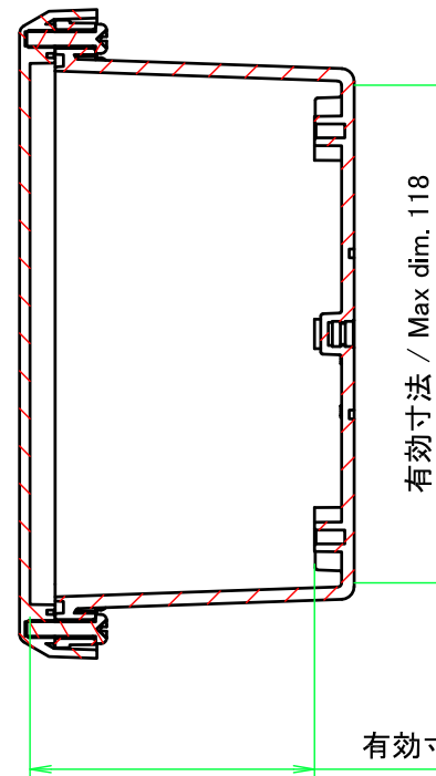
A-A ( 1 : 2 )
