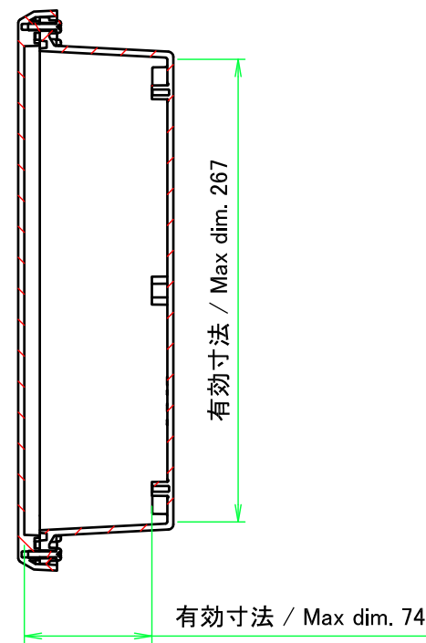
A-A (1:4)
