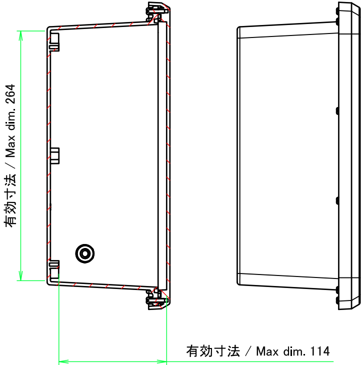
A-A (1:4)
