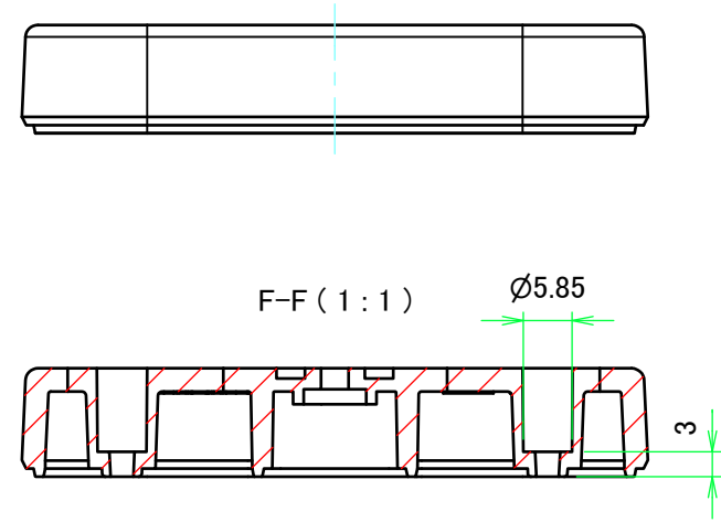
ポールマウントブラケット (WPMB-M3) 用取付ガイド Mounting position for Pole Mounting Bracket (WPMB-M3)
