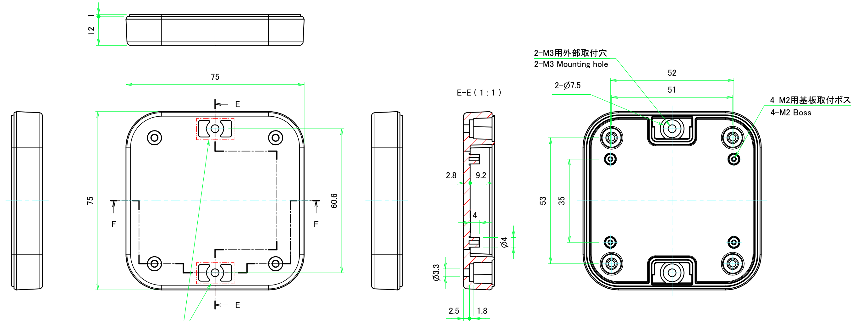
ポールマウントブラケット (WPMB-M3) 用取付ガイド Mounting position for Pole Mounting Bracket (WPMB-M3)
