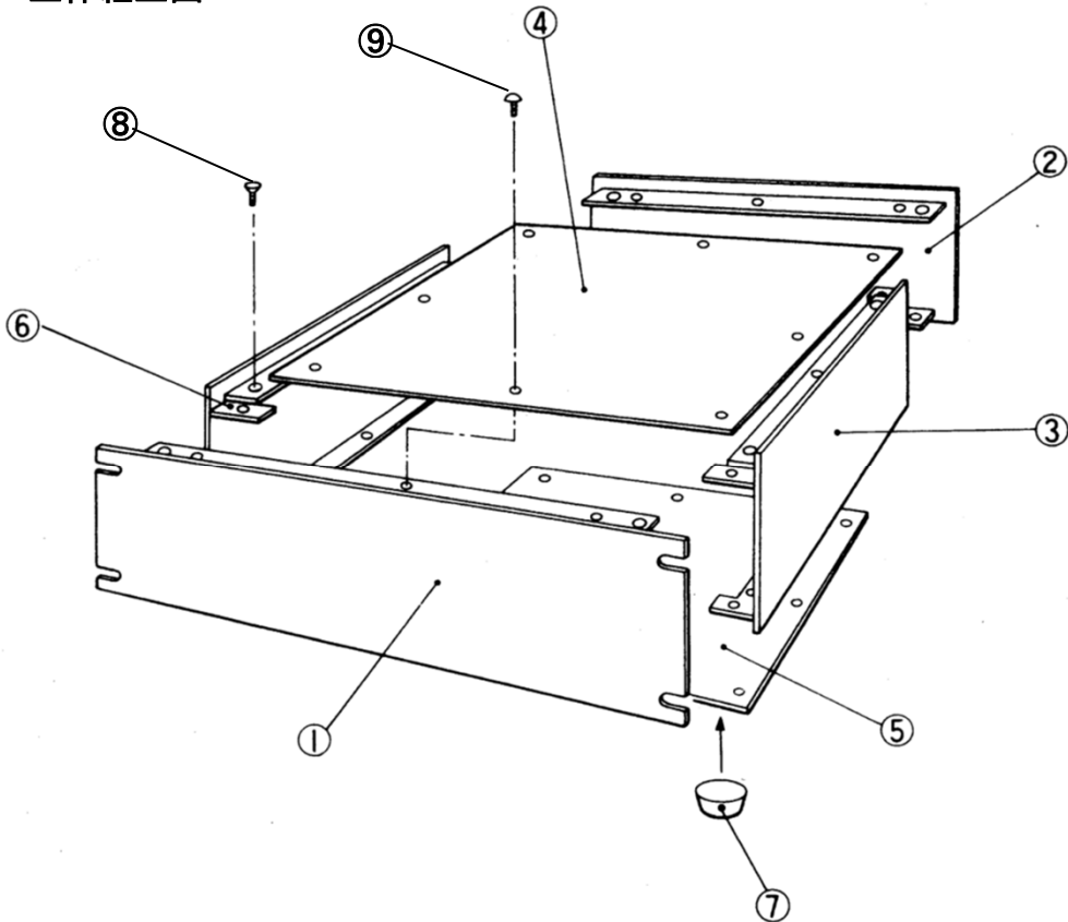
立体組立図
