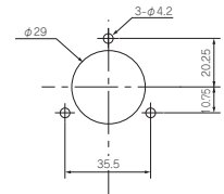
取付け穴寸法
