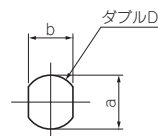
取付穴寸法図
