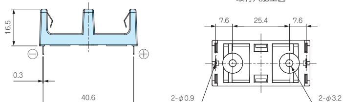
取付穴加工図
