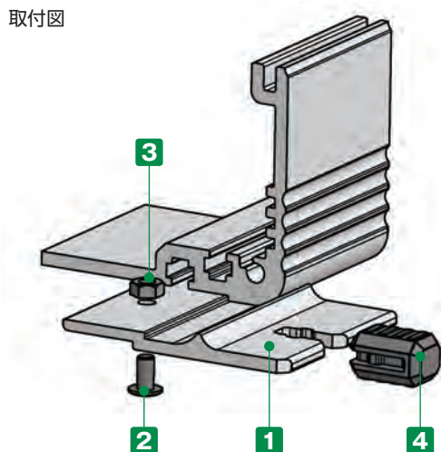
取付図
