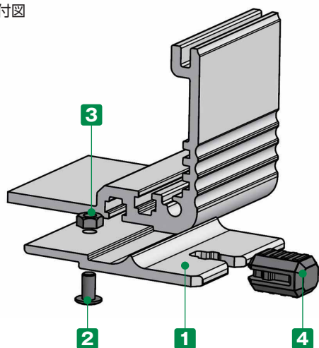
取付図
