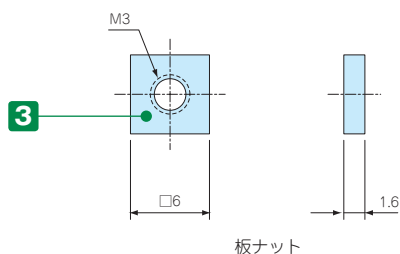
板ナット
