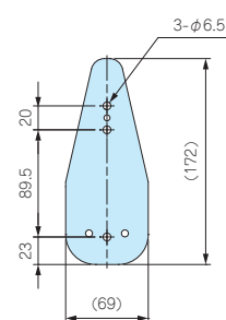
壁付ブラケット寸法
