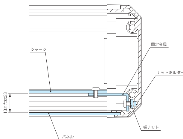
取付図
