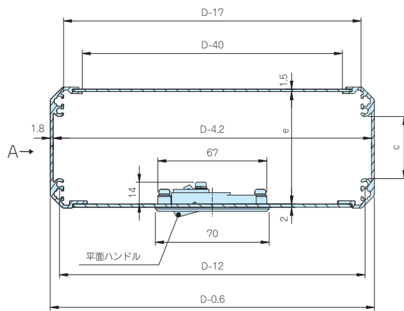
D方向図
