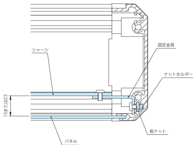
取付図
