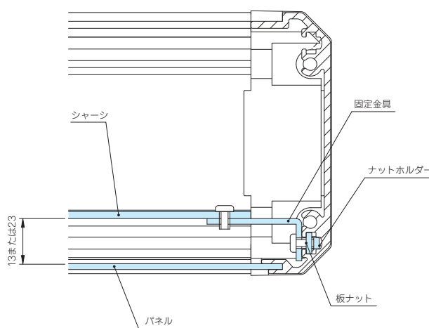
取付図
