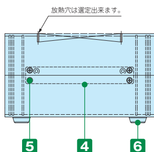
シャーシ UCSCシリーズ P10-135
