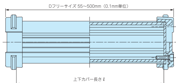
D寸法
