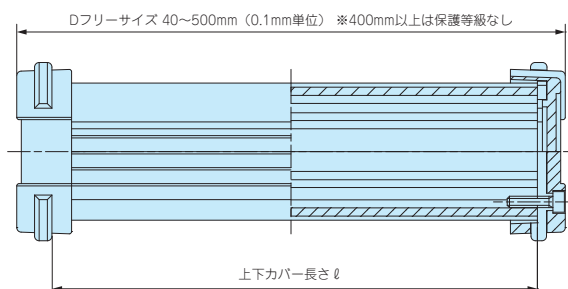
D寸法
