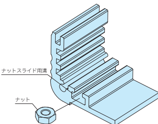
スライド溝用ナット MT-3N P10-107
