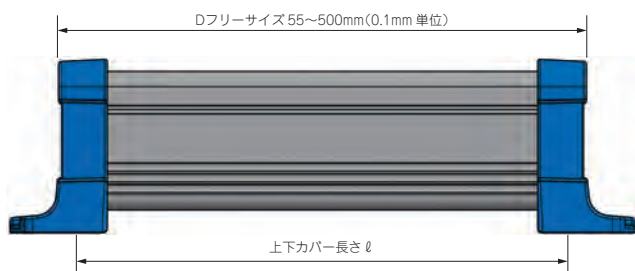
D寸法
