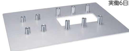
パネル穴加工+クリンチングスペーサー 実働6日目発送
