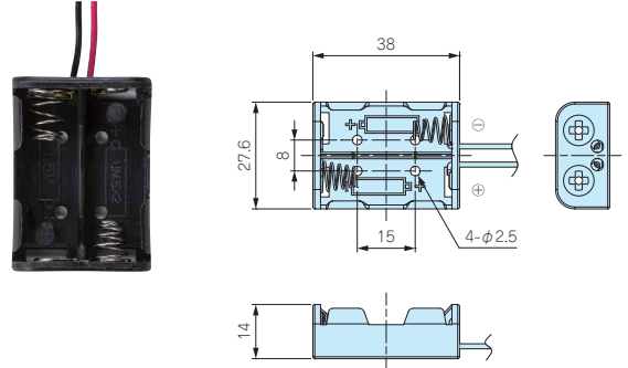
BH-521A 単5×2本
