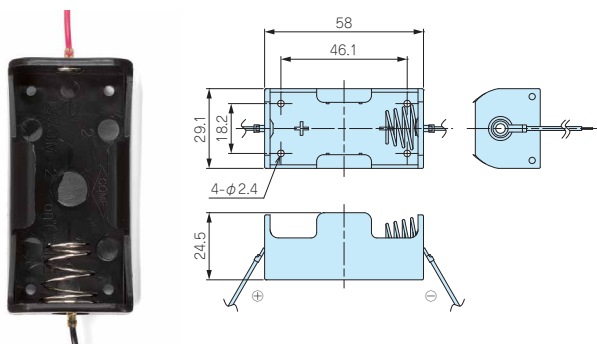
BH211-1 単2×1本
