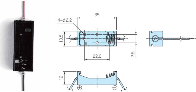
MP-5-1N 単5×1本
