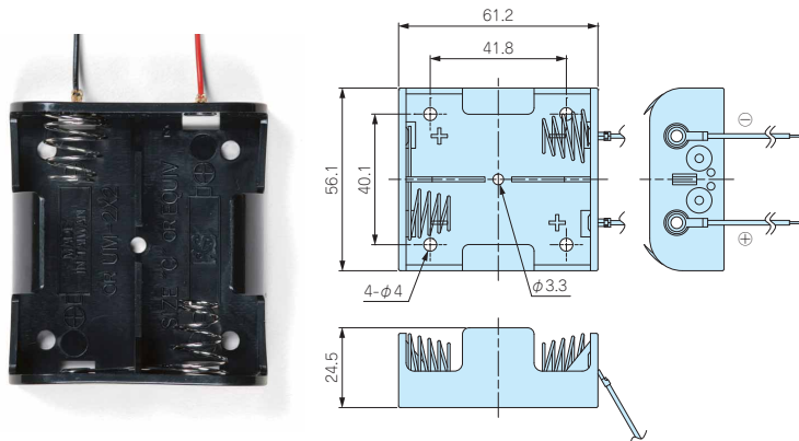
SN 2-2 単2×2本
