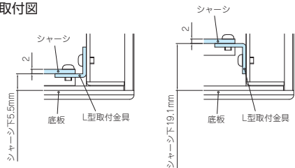
取付図
