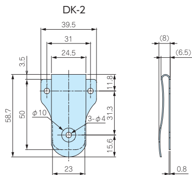
取付穴寸法図
