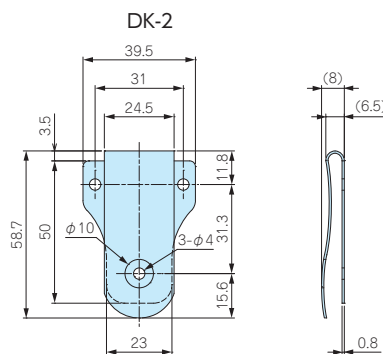
取付穴寸法図
