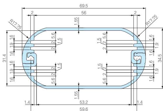
MXAC/MXC70-35-□
