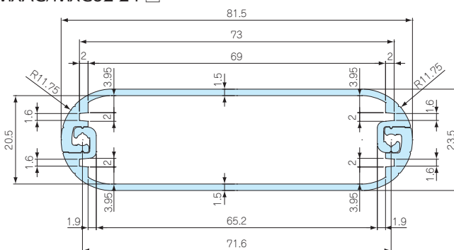
MXFC86-30-□ MXAC/MXC82-24-□
