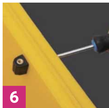
ドライバーでしっかりビスを締める。 (締付トルク値 0.8~1.0N・m)
