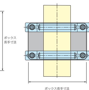
よこ型取付 (長手寸法よこ)
