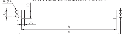
取付穴寸法図 (取付部推奨板厚: 2.0mm)
